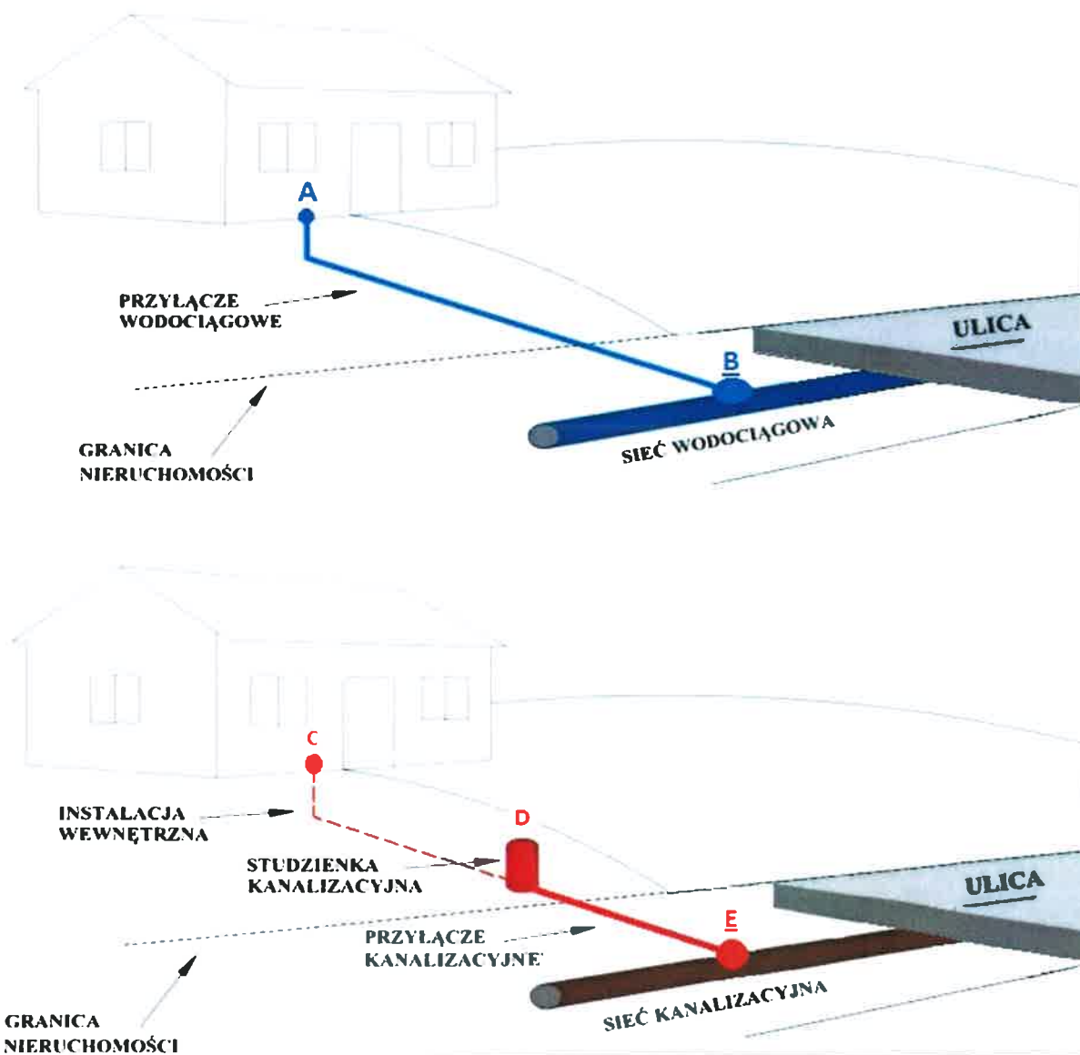
Szkic sytuacyjny
