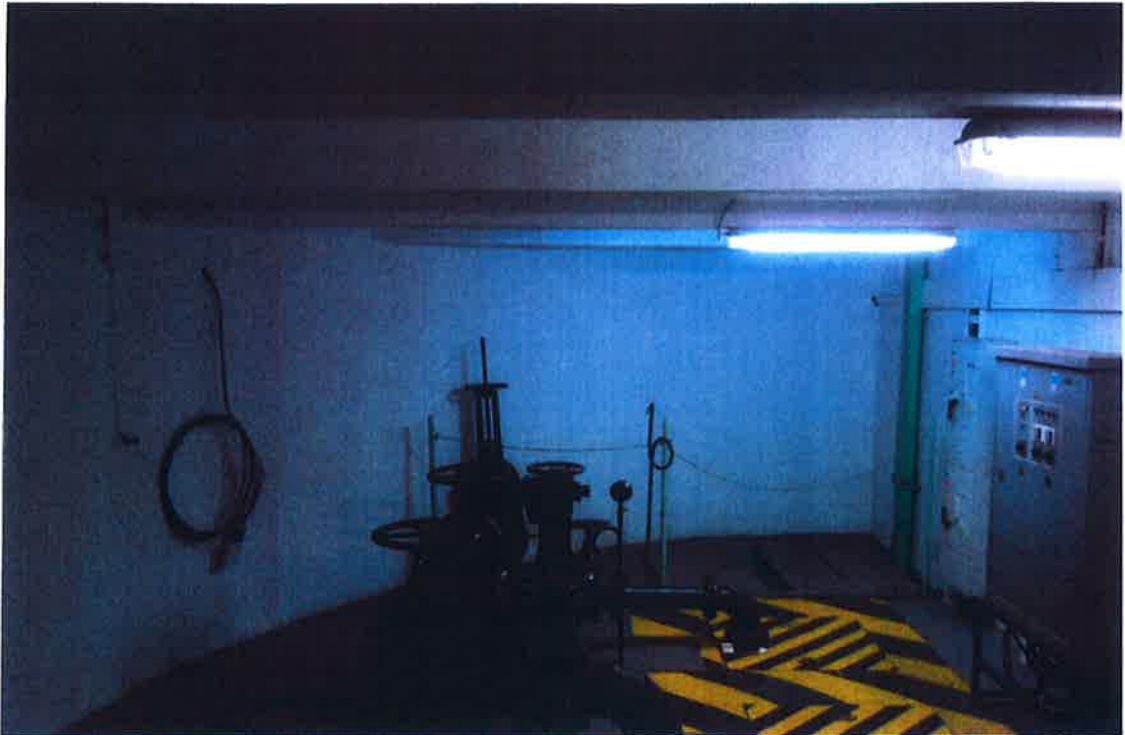
Pompownia centralna – komora zasuw
